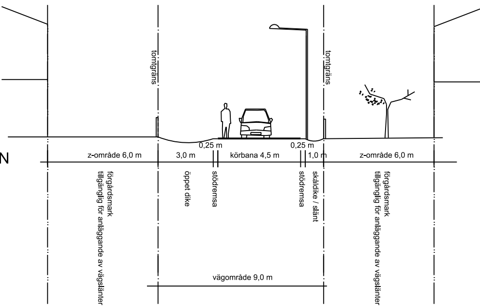
Sektion vid fastigheten 1:117
