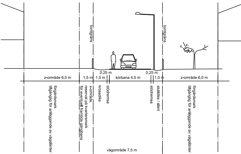
Sektion vid fastigheterna 1:691 och 1:692
