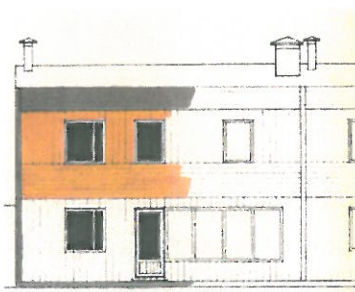
Hustyp S2, entré- och gårdsfasad
