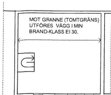
PÅBYGD VÅNINGSPÅN SKALA 1:200
