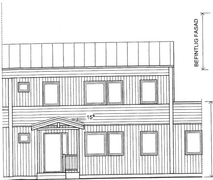
NY FASAD SKALA 1:100
