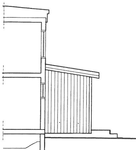
SEKTION/FASAD
