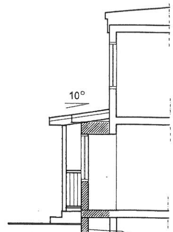
SEKTION/FASAD
