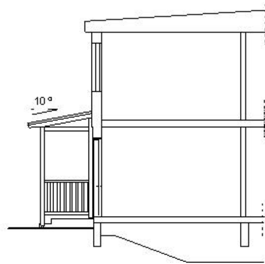
SEKTION ALT 2
