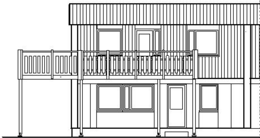
FASAD
