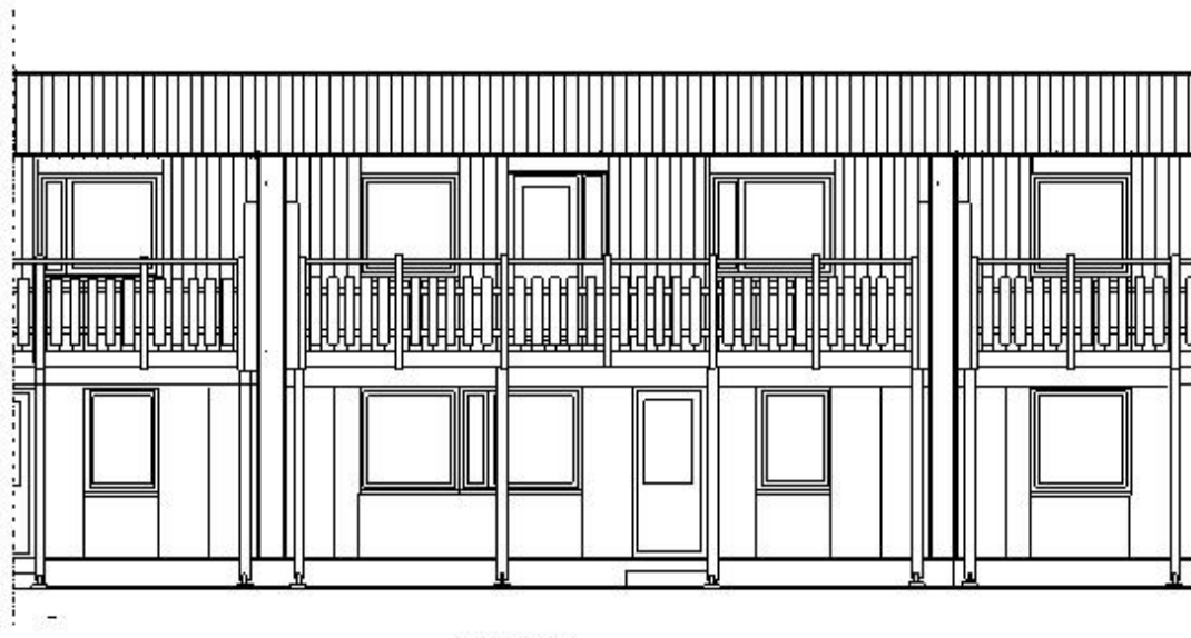
FASAD
