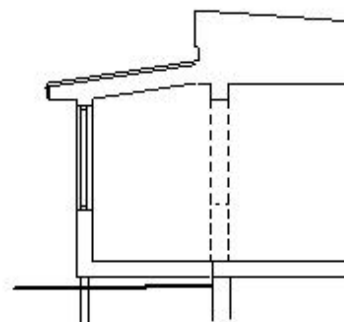
SEKTION BURSPRÄK
