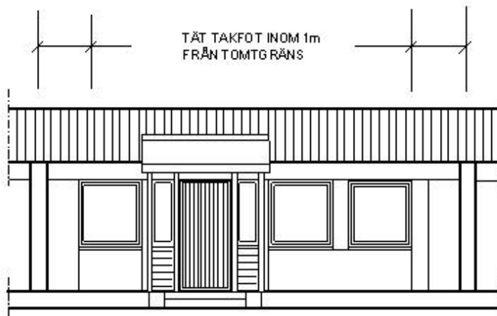
FASAD FÖRSTUKVIST TYP 2
