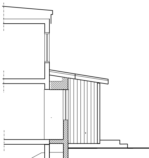
SEKTION / FASAD
