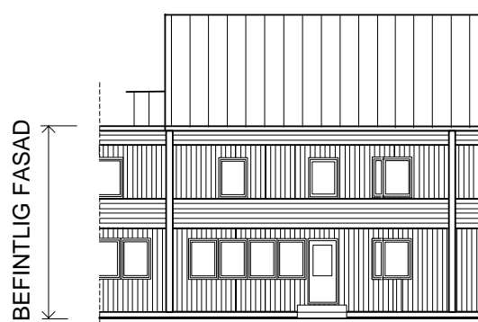
SKALA 1:200
