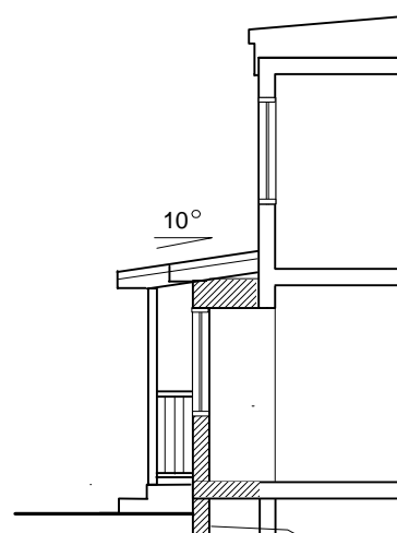
SEKTION/FASAD
