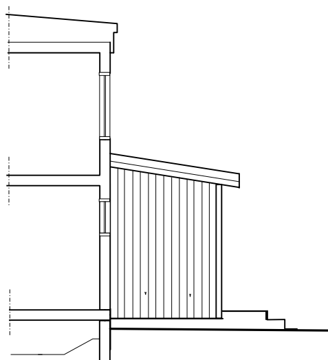
SEKTION/FASAD
