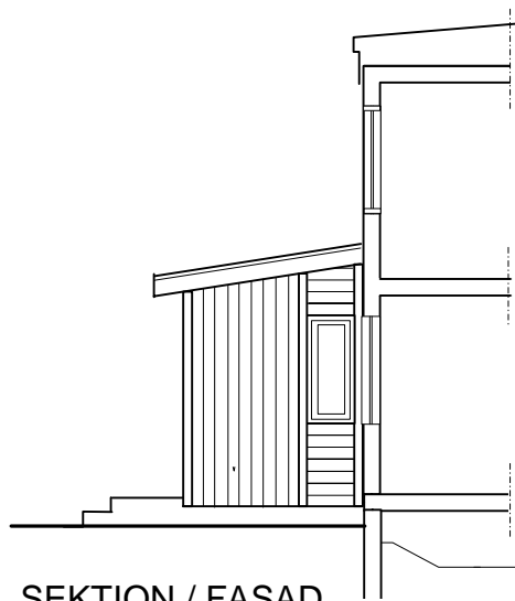
SEKTION / FASAD
