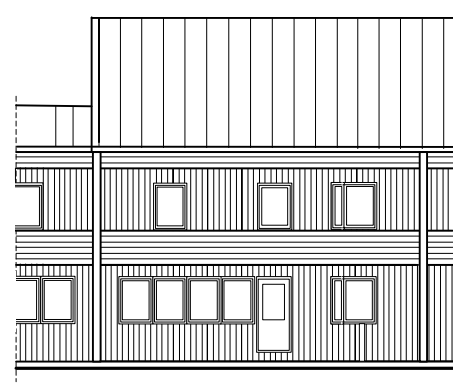
SKALA 1:200
