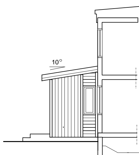
SEKTION/FASAD
