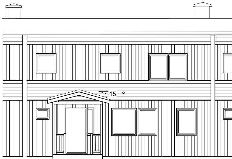
FASAD
