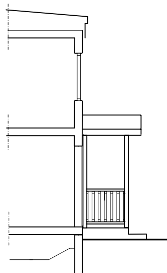
SEKTION/FASAD
