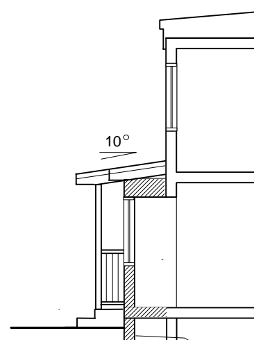
SEKTION/FASAD
