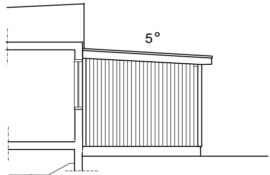
SEKTION / FASAD
