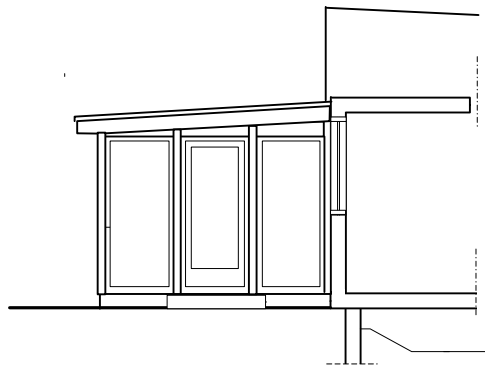
SEKTION / FASAD
