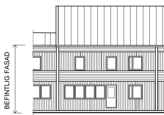
SKALA 1:200
