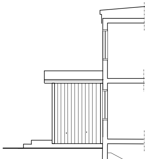
SEKTION / FASAD
